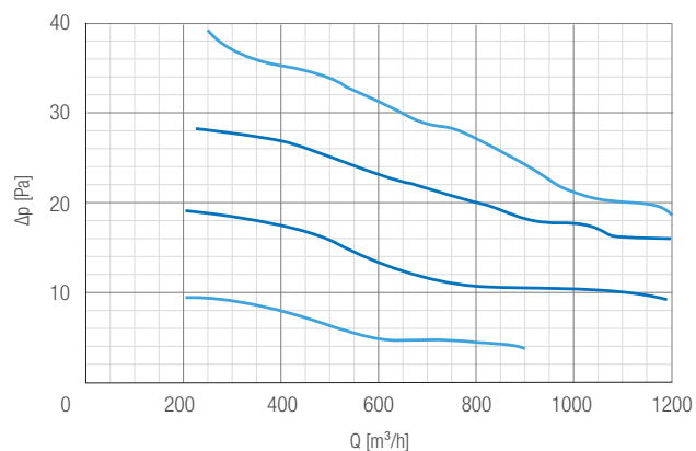
Charakterystyki przepływowe
